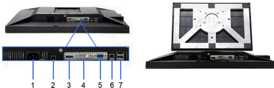
底视图
